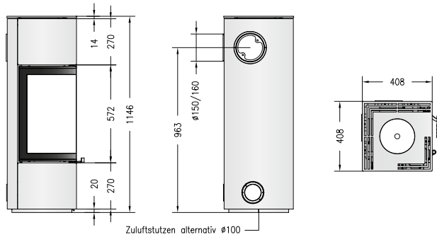
Maße der feststehenden Variante
